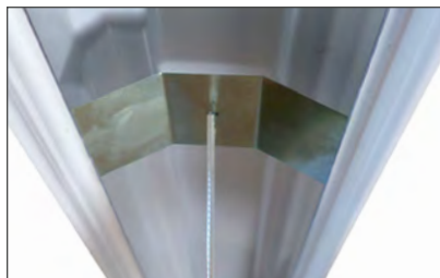
Montagehilfe/Sicherungsclip aus Federstahl lässt sich einfach in die Tragschiene einclippen.
